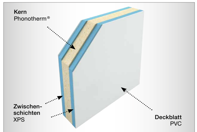
thermische Konstruktionsplatte, Verstärkung Rollkastensysteme
