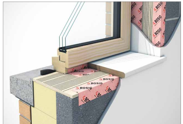
Trägerplatte bei Fensterunterkonstruktion
